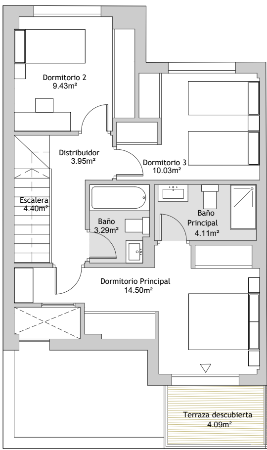
PLANTA PRIMERA
