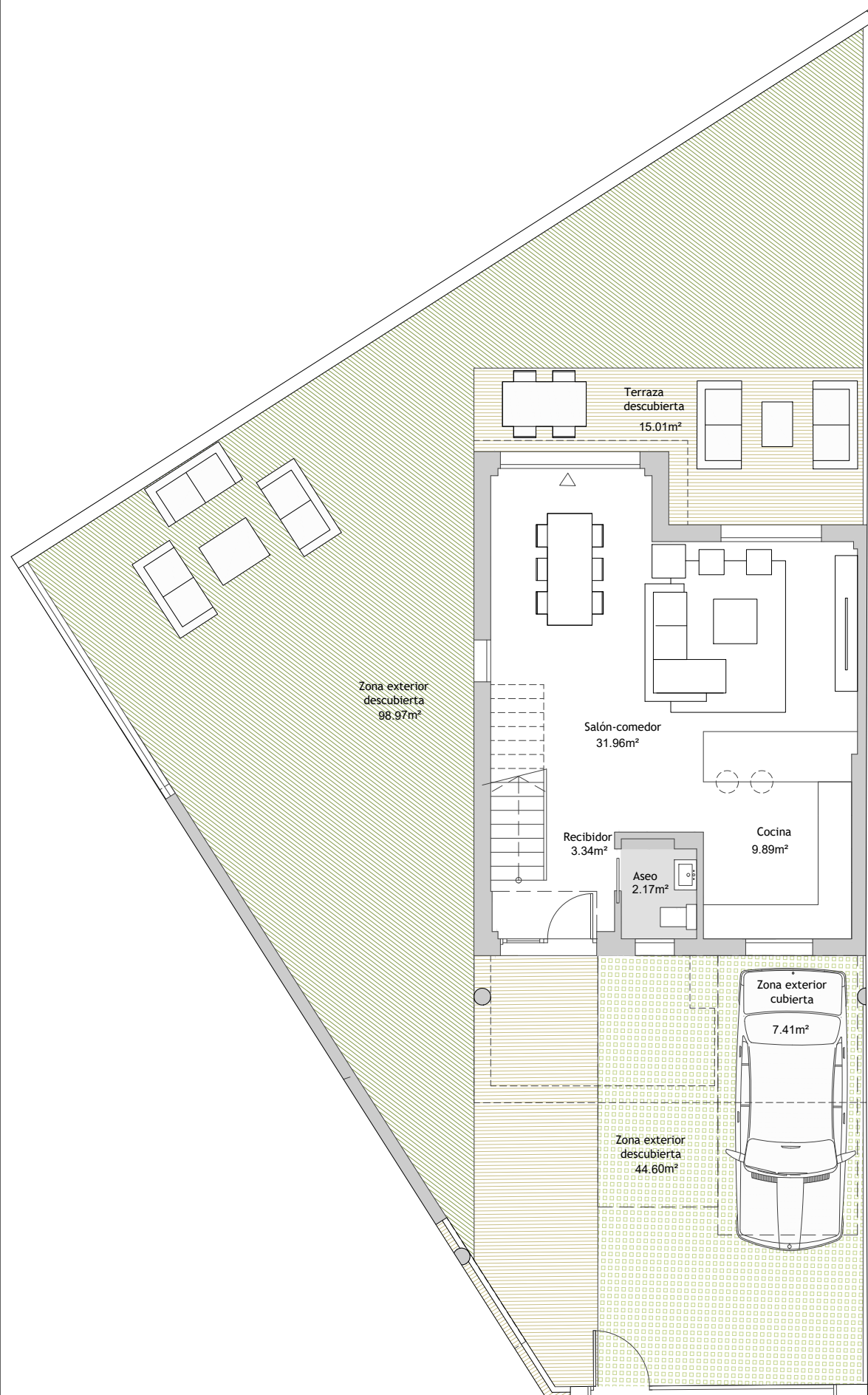
PLANTA BAJA
