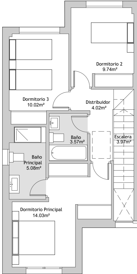
PLANTA PRIMERA
