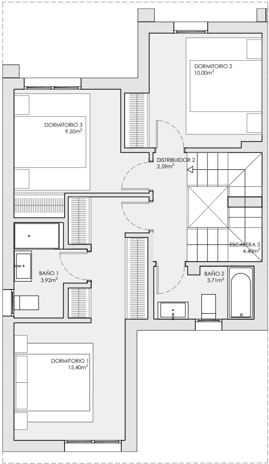
PLANTA PRIMERA
